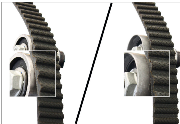
Billede 2: Afbøjningsremskive 532 0623 10 (venstre)/afbøjningsremskive 532 0349 10 (højre)
