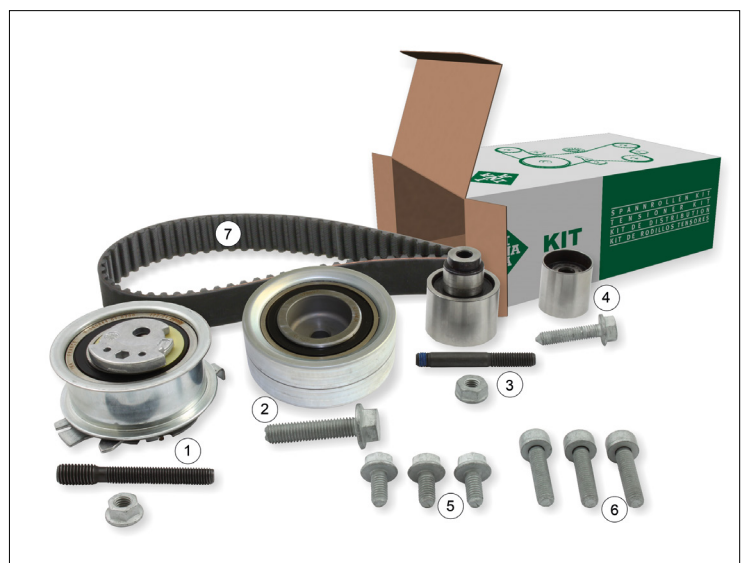
Slika 1: Kat. Br. 530 0550 10 INA Kit natezne remenice
