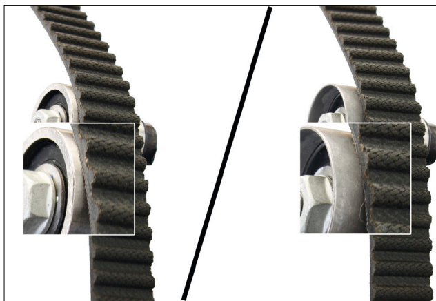
Рисунок 2: Направляющий ролик 532 0623 10 (слева)/направляющий ролик 532 0349 10 (справа)
