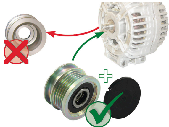
Εικόνα 1: Αλλάζοντας μια συμπαγή τροχαλία σε μία τροχαλία με κασάνια
