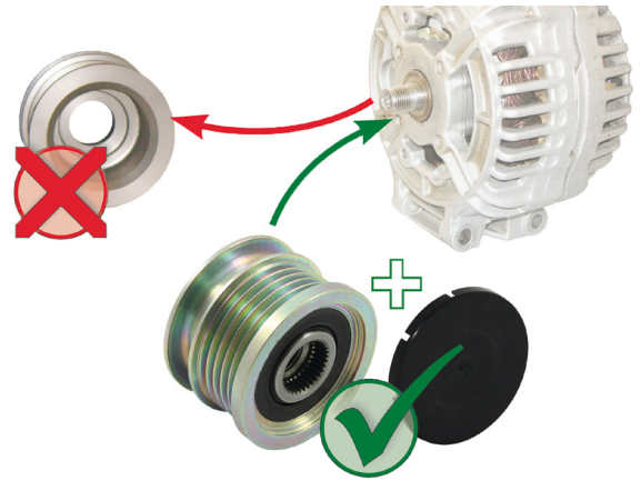
Kuva 1: Kiinteän hihnapyörän vaihto laturin vapaapyörään
