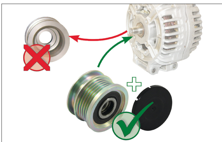
Slika 1: Zamjena krute remenice sa remenicom slobodnog hoda alternatora
