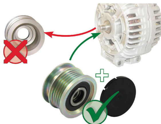
Figura 1: Schimbarea unei fulii de curea rigide la o folie de alternator cu ambreiaj de mers liber
