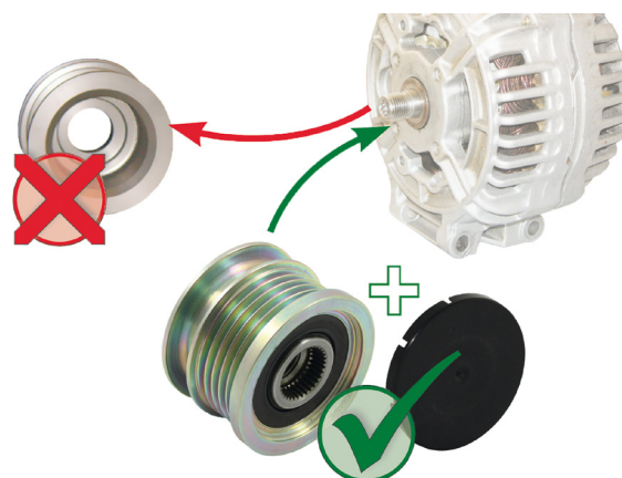
Bild 1: Utbyte av fast remskiva mot generatorfrinav
