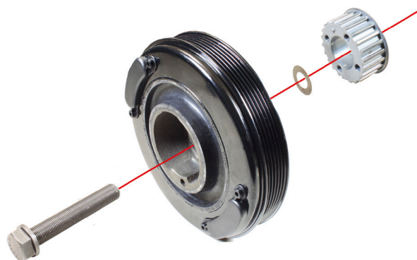
Sada řemenice 544 0002 20 se skládá z tlumiče vibrací klikové hřídele s centrálním šroubem klikové hřídele a podložky pokryté diamanty
