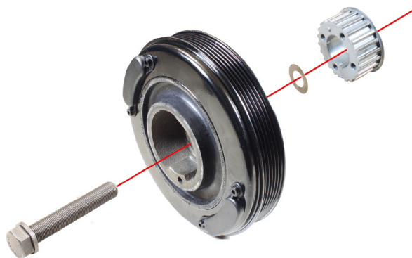
Figur 1: veivaksels vibrasjonsdemper med sentral skruer til veivaksel og diamantskive
