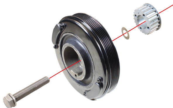
Remskivesatsen 544 0002 20 består av vibrationsdämpare för vevaxeln med vevaxelskruv och en diamantbelagd bricka
