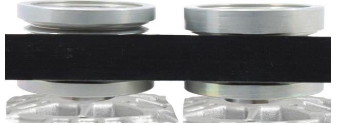
Resim 1: Sol: 6 kanallı 535020210 INA devir ayarlı alternatör kasmağı - Sağ: 5 kanallı INA devir ayarlı alternatör kasmağı
