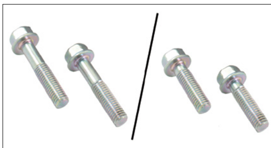
Fig 4: Links, oude bouten M8x40 mm Rechts, nieuwe bouten M8x30 mm
