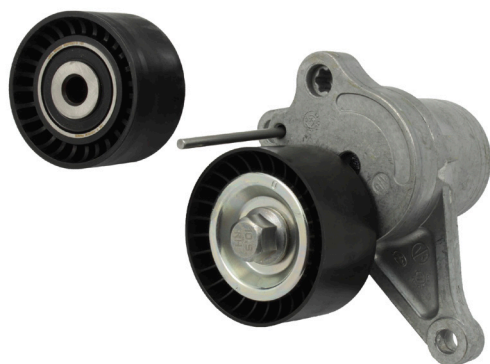
Εικόνα 2: Πλαστική τροχαλία τένυσης και τροχαλία εκτροπής
