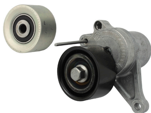
Εικόνα 1: Μεταλλική τροχαλία τένυσης και τροχαλία εκτροπής
