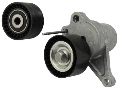
2. ábra: Műanyag feszítő- és vezetőgörgő
