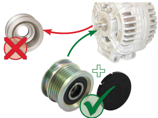
Εικόνα 1: Αντικαθιστώντας μια άκαμπτη τροχαλία ιμάντα με μια τροχαλία δυναμό με κασάνια
