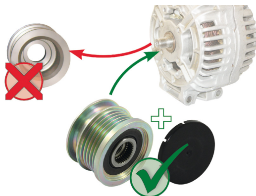
Figur 1: Skifte fra en stiv remskive til en friløpsremskive OAP
