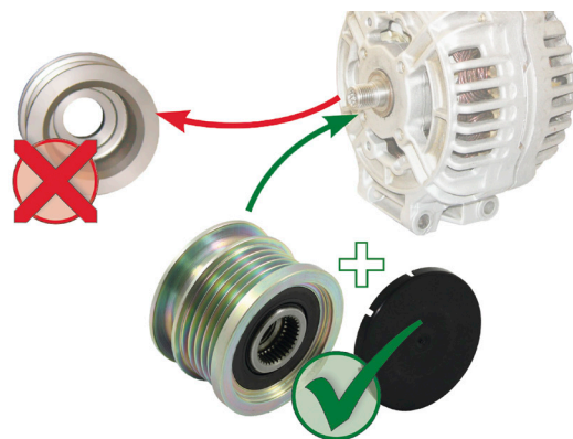
Рисунок 1: Замена жесткого шкива на шкив генератора с обгонной муфтой
