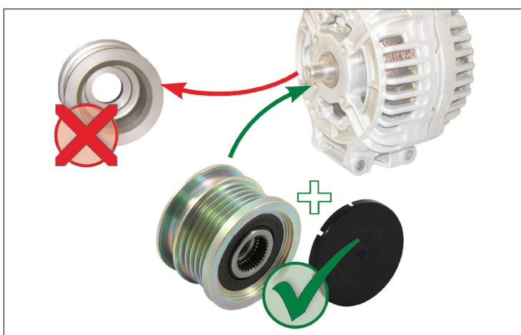
Slika 1: Prehod s toge jermenice na jermenico alternatorja s sklopko za prosti tek
