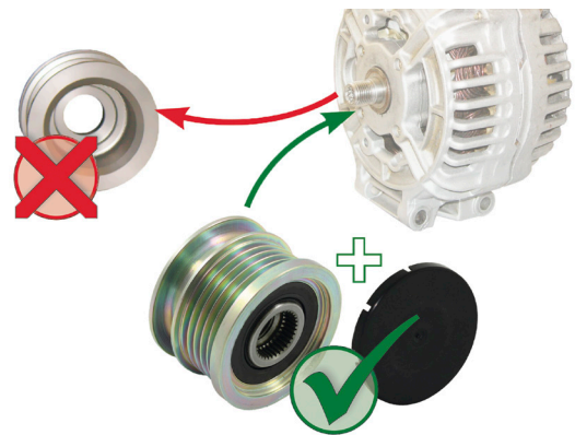
Зображення 1: Заміна жорсткого шків на шків генератора з обгінною муфтою
