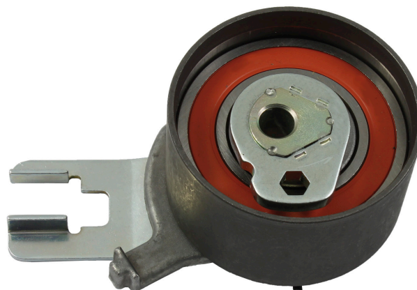
Рисунок 2: 531 0515 10 – натяжной ролик прежней конструкции.
