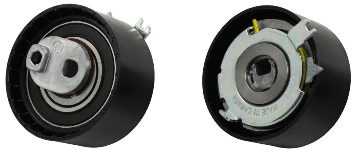
Bild 1: INA-Spannrolle 531 0710 10
