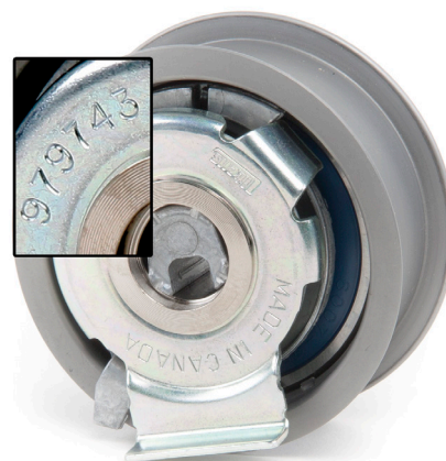
Obr. 1: 531 0777 10 – stará napínací kladka (979743)
