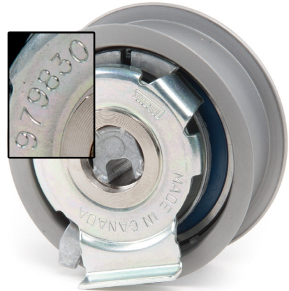
Kuva 2: 531 0851 10 – uusi hihnankiristin (979830)
