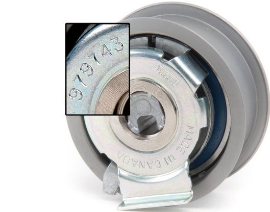
Kuva 1: 531 0777 10 – vanhaa hihnankiristin (979743)
