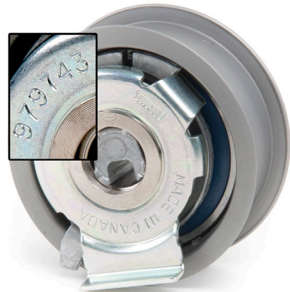
1. ábra: 531 0777 10 – régi feszítőgörgő (979743)
