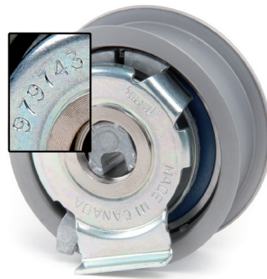
Fig. 1: 531 0777 10 – oude spanrol (979743)
