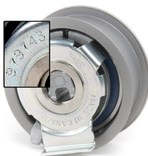
Slika 1: 531 0777 10 – prejšnja napenjalna jermenica (979743)
