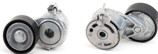
Рисунок 2: Новая конструкция
