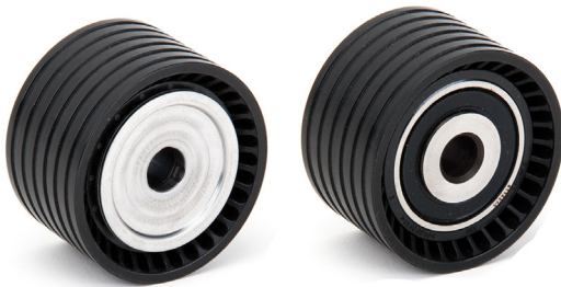
Kuva 1: Ohjainpyörät vanhalla tiivistekonseptilla
