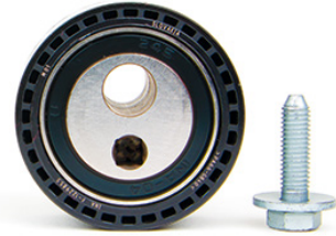
Kuva 3: 531 0264 10 - INA-kiristinpyörä ruuvilla
