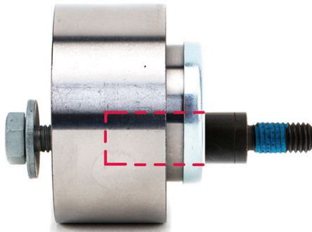
איור 4: גלגלת מותחן בעלת שרוול הברגה ובורג הידוק כאשר היא מותקנת למקומה
