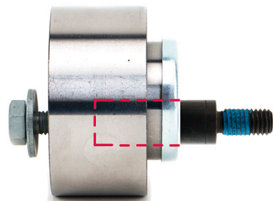
4. ábra: INA feszítőgörgő hüvelyes és rögzítőcsavarral a beszerelési helyzetben
