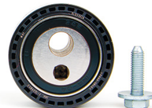
Bild 3: 531 0264 10 - spännrulle från INA med medlevererad skruv
