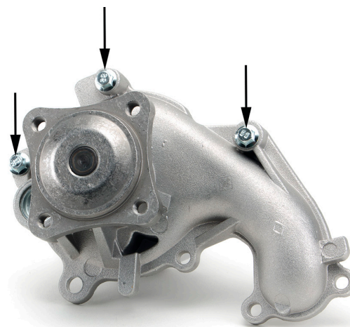
Obrázek 2: Modifikované upevňovací body čerpadla chladicí kapaliny
