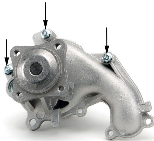
Εικόνα 2: Διαφοροποιημένα σημεία στήριξης της αντλίας νερού
