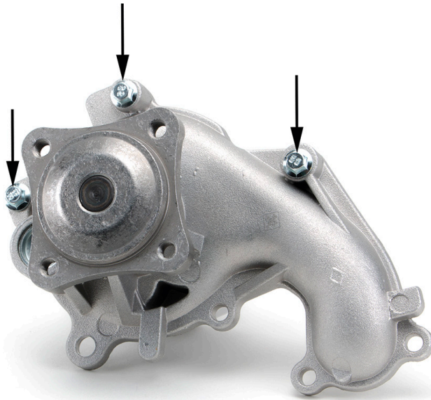
תמונה 2: נקודות בהן בוצע השיפור על משאבת המים
