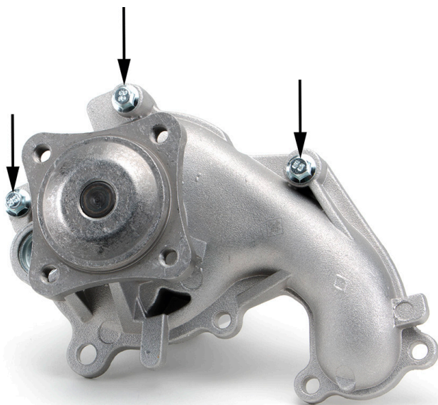
Slika 2: Modificirani provrti za učvršćenje vodene pumpe – označeni strelicama
