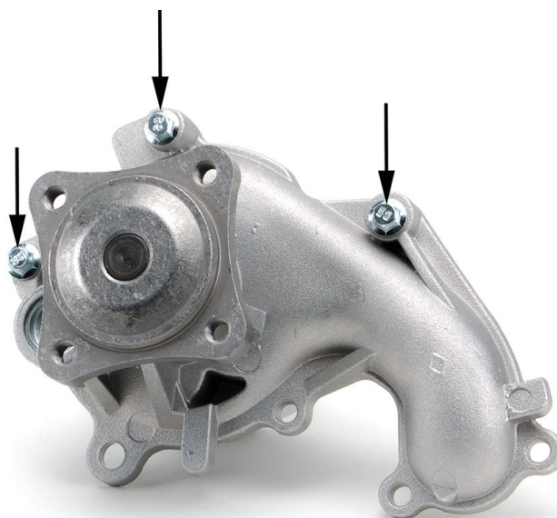
Fig. 2: Pontos de fixação modificados da bomba de refrigerante
