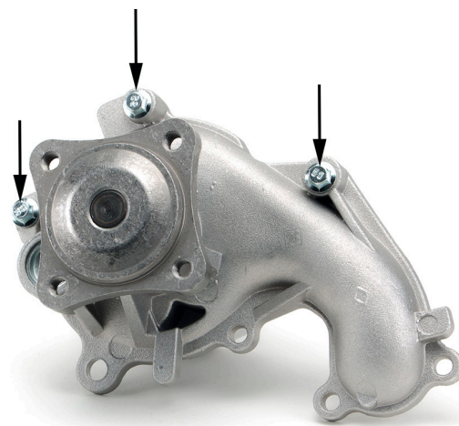
Рисунок 2: Измененные кронштейны креплений водяного насос
