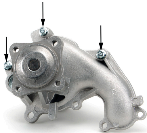
Зображення 2: Модифіковані місця для кріплення насоса охолоджувальної рідини
