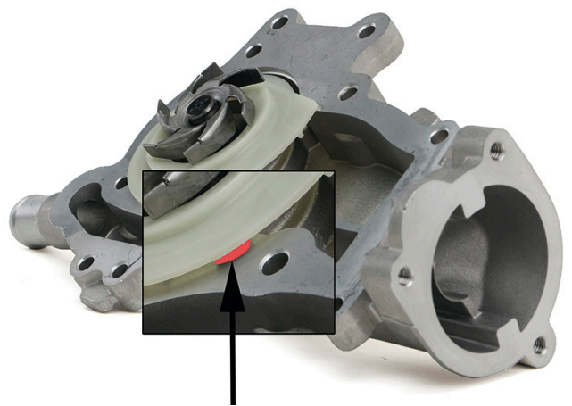
Зображення 2: Послаблена пластмасова прокладка через надлишок герметика
