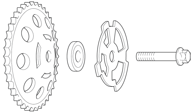
Kuva 2: Oikea asennusjärjestys imupuolen nokka-akselissa vaihdettaessa sintratusta materiaalista tehty ketjupyörät puristettuihin.
