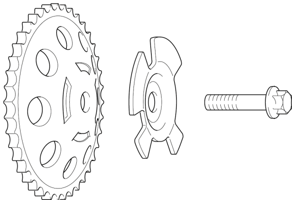
תמונה 4: מראה של מצב התקנה נכון על גל הזיזים אשר בצד היניקה לאחר החלפת גלגל שיניים אשר מיוצר ממתכת בלחיצה.
