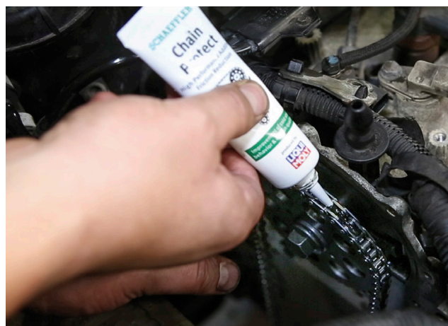
Снимка 2 Schaeffler Chain Protect се прилага за всички компоненти на ангренажната веригата по време на монтажа.
