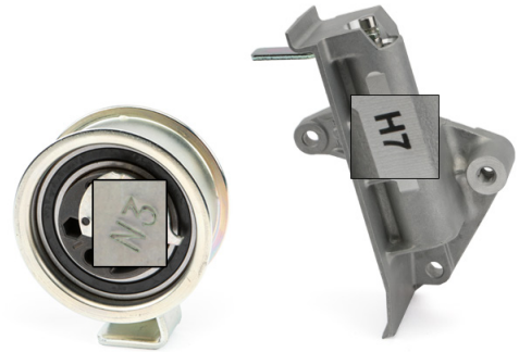
Kuva 1: Kiristinpyörä 531 0396 20 ja värinänvaimennin 533 0039 10
