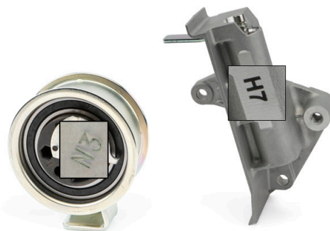
1. ábra: 531 0396 20 cikkszámú feszítőgörgő az 533 0039 10 cikkszámú rezgéscsillapítóval
