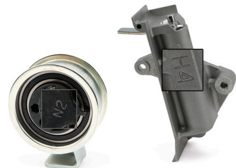
2. ábra: 531 0436 20 cikkszámú feszítőgörgő az 533 0035 10 cikkszámú rezgéscsillapítóval
