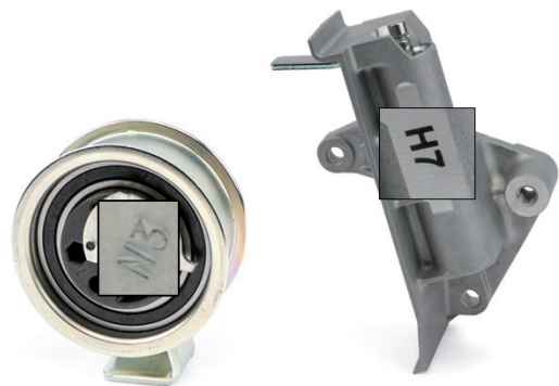
Afbeelding 1: Spanrol 531 0396 20 met trillingsdemper 533 0039 10
