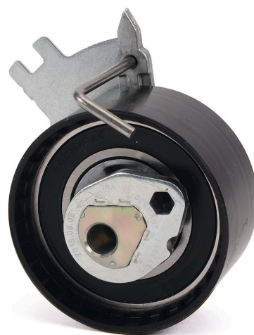
Зображення 2: Модифікований натяжний ролик 531 0885 10
