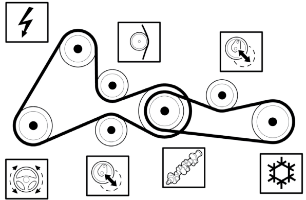
Kuva 1: Apulaitekäyttö moottorin numeroon 0113089 saakka kiristinpyörällä
