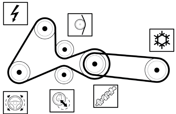
Kuva 2: Apulaitekäyttö moottorin numerosta 0113090 alkaen elastisella moniurahihnalla
