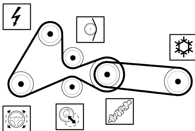
Slika 2: Shema razvoda pogona pomoćnih agregata s elastičnim kanalnim remenom; od serijskog broja motora 0113090
